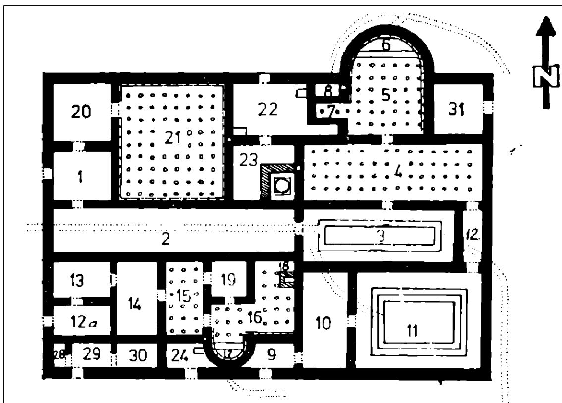
Figura 29. Planul clădirii EM 25 (după P. Király)
